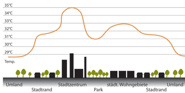
Temperaturverlauf der städtischen Hitzeinsel vom Stadtrand zum Zentrum
